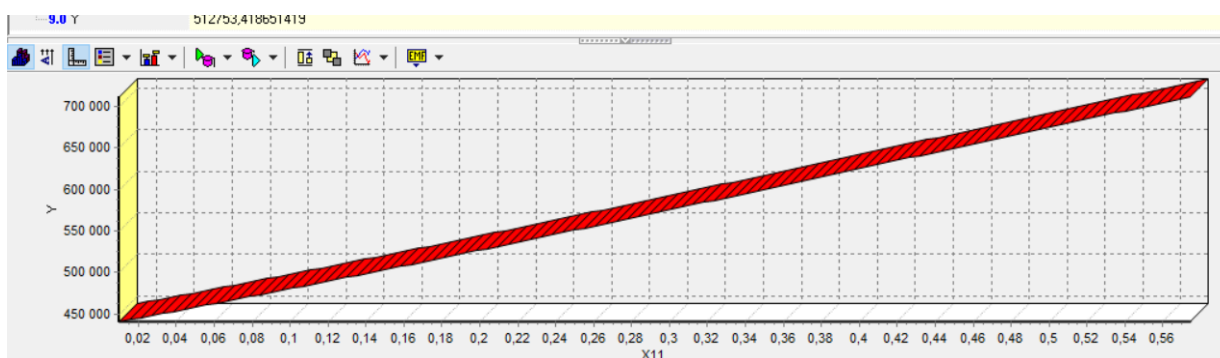
Рис. 6. График зависимости Y от X11 для Волгоградской области в 2021 г.
