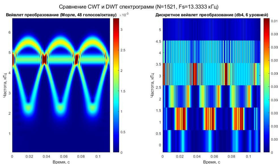
Рис. 5. Спектрограммы непрерывного и дискретного вейвлет преобразования
