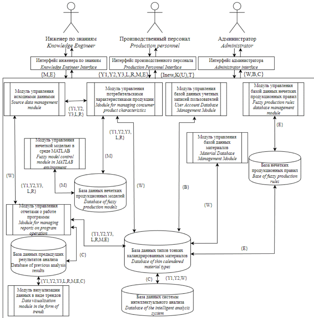
Рис. 6. Функциональная структура программного комплекса
