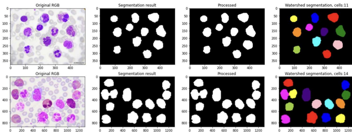
Рис. 4. Иллюстрация промежуточных результатов этапа постобработки бинарной маски Fig. 4. Illustration of intermediate results of the binary mask post-processing stage
