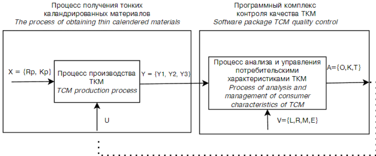
Рис. 4. Формализованное описание процесса управления качеством ТКМ Fig. 4. Formalized description of the TCM quality management process
