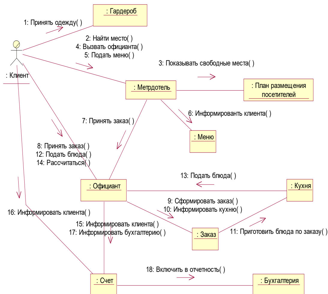
Рис. 2. UML-диаграмма взаимодействия объектов (кооперации) для прецедента «Обслуживаниеобеда/ужина» как часть О-модели деятельности ресторана Fig. 2. UML-diagram of object interaction (cooperation) for the “Lunch/Dinner Service” use case as part of the O-model of restaurant activities
