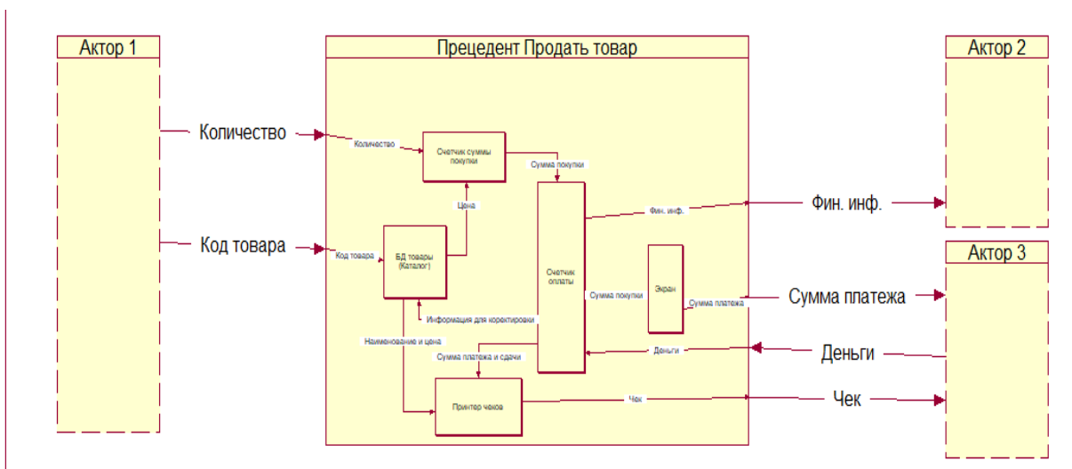
Рис. 7. УФО-диаграмма прецедента «Продать товар» Fig. 7. UFO-diagram of the “Sell a product” use case
