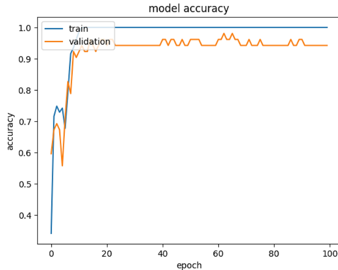
Рис.10. Результат обучения GRU модели ИНС Fig.10. Result of training GRU ANN model
